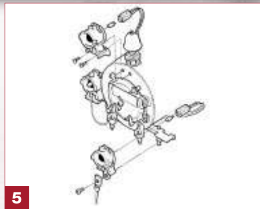
Lampen vorne
