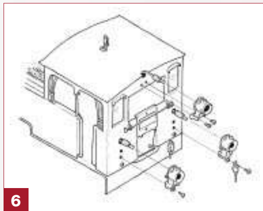
Lampen hinten
